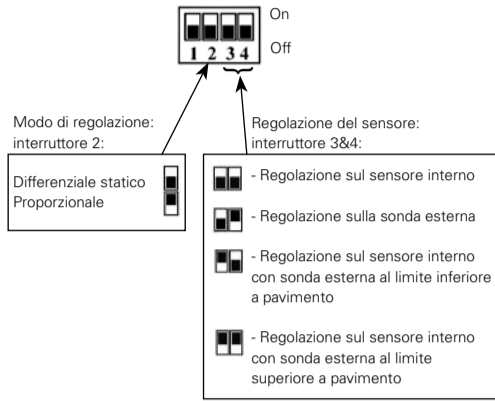
RTS01 Sensore esterno opzionale 10K
