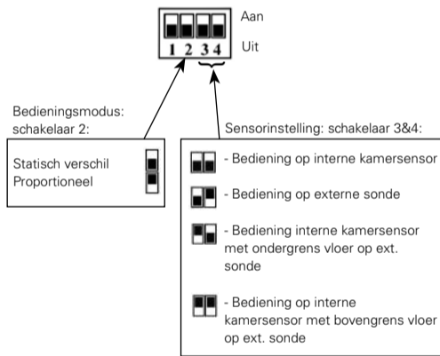
RTS01 Optionele externe sensor 10K
